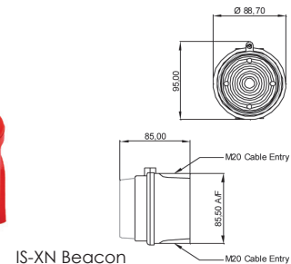
IS-XN Beacon
